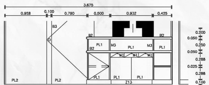
ALZADO A MSD-32 VER P. CA-07B-11
