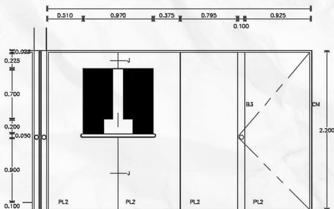
ALZADO B MSD-32 VER P. CA-07B-11
